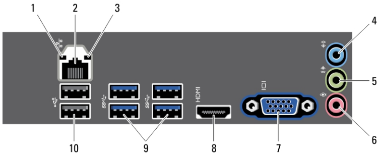
그림 2. 후면 패널 모습
